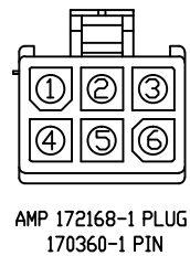
MOTOR CONNECTOR 접속도
