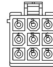
ENCODER 접속도
