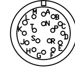
MS3102A20-29P Encoder Cable Connector 접속도
