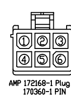
MOTOR CONNECTOR 접속도
