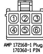
MOTOR CONNECTOR 접속도
