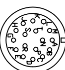
MS3102A20-29P Encoder Cable Connector 접속도
